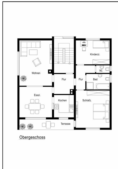
Grundriss Obergeschoss
